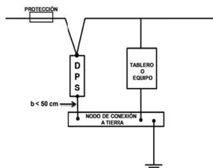
Figura 20.2 Montaje típico de DPS
