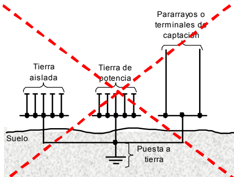
Figura 15.2. Puestas a tierra separadas o independientes
