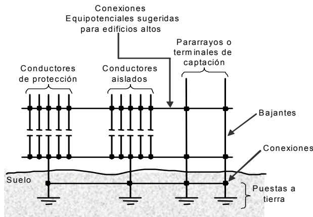
Figura 15.1. Sistemas con puestas a tierra dedicadas e interconectadas
