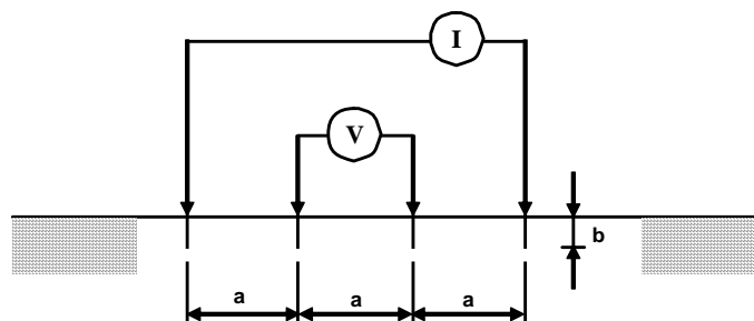
Figura 15.4. Esquema de medición de resistividad aparente
