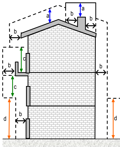
Figura 13.1. Distancias de seguridad en zonas con construcciones
