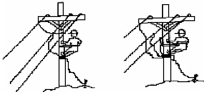
Figura 15.6. Montajes típicos de puestas a tierra temporales
