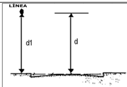
Figura 13.2. Distancias "d" y "d1" en cruce y recorridos de vías
